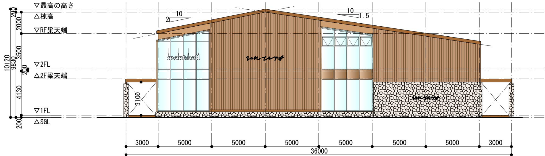
[南側立面図]
