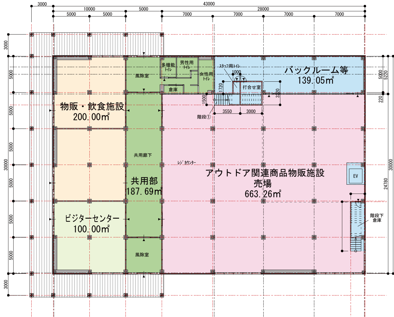
1階平面図
