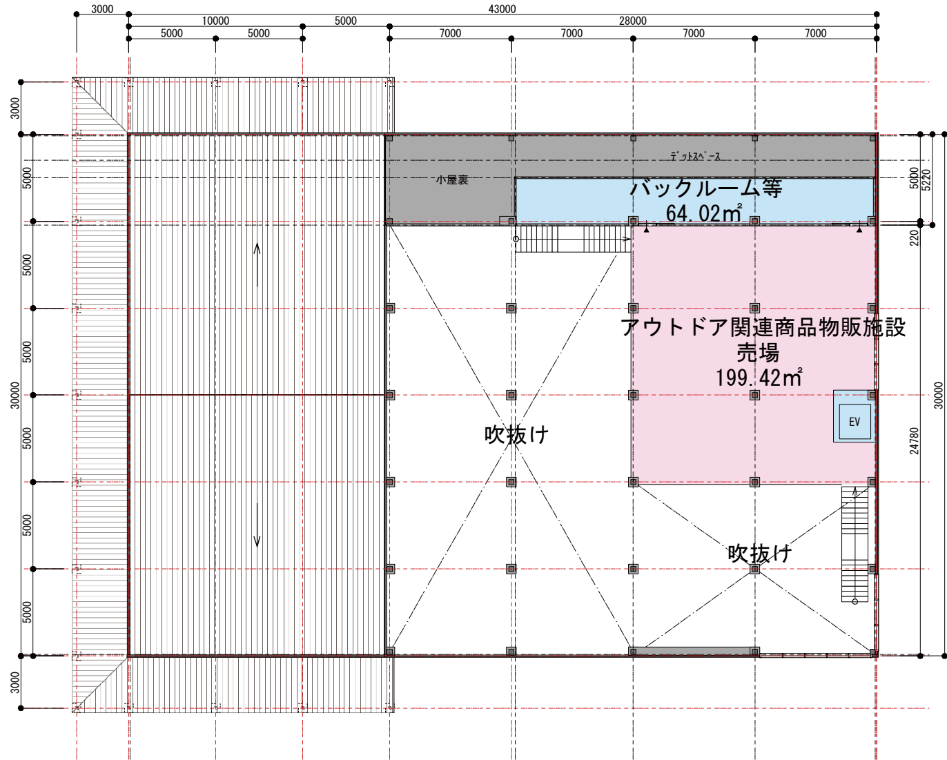
2階平面図
