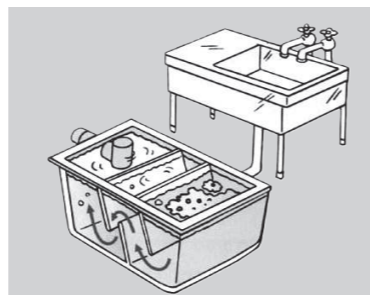
▲飲食店などのグリーストラップ
