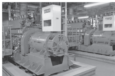
▲留萌市立病院の非常用自家発電設備
