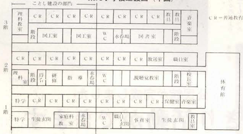
東光小学校建設図(平面)
