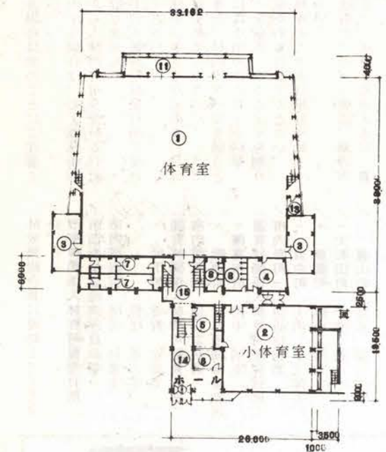
2階平面図
