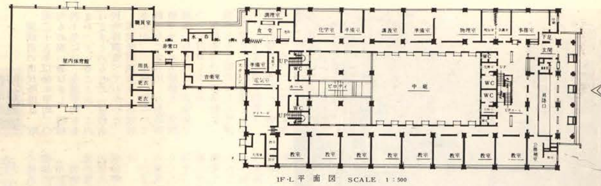
1F-L 平面図 SCALE 1:500
