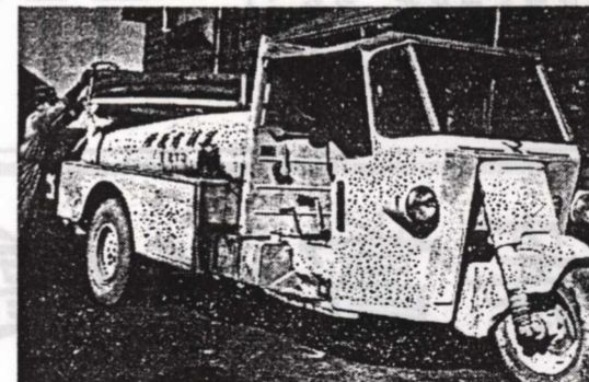
汚物処理に威力を加えた小型尿処理タンク車。積載量は十石です
