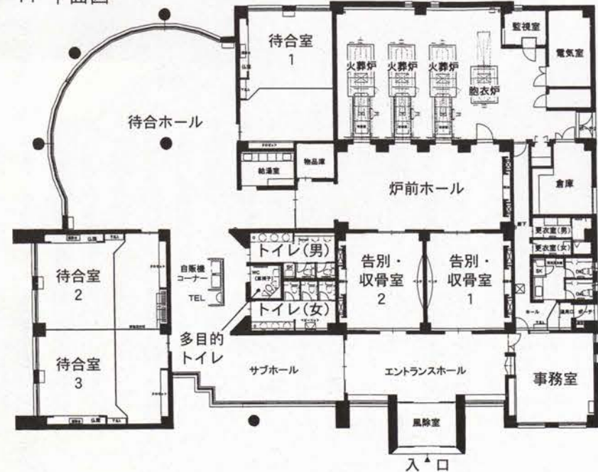
1F 平面図
